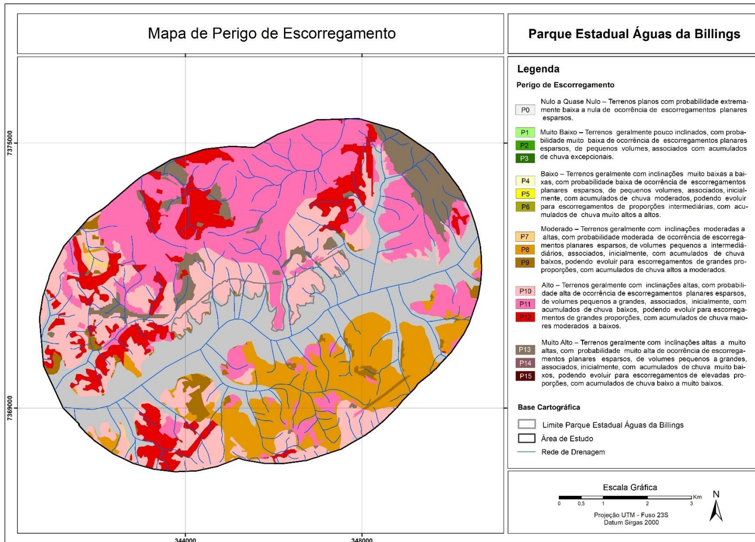
APÊNDICE 3.7.F Mapa de Perigo de Escorregamento Planar da área de estudo. Fonte: autores.
