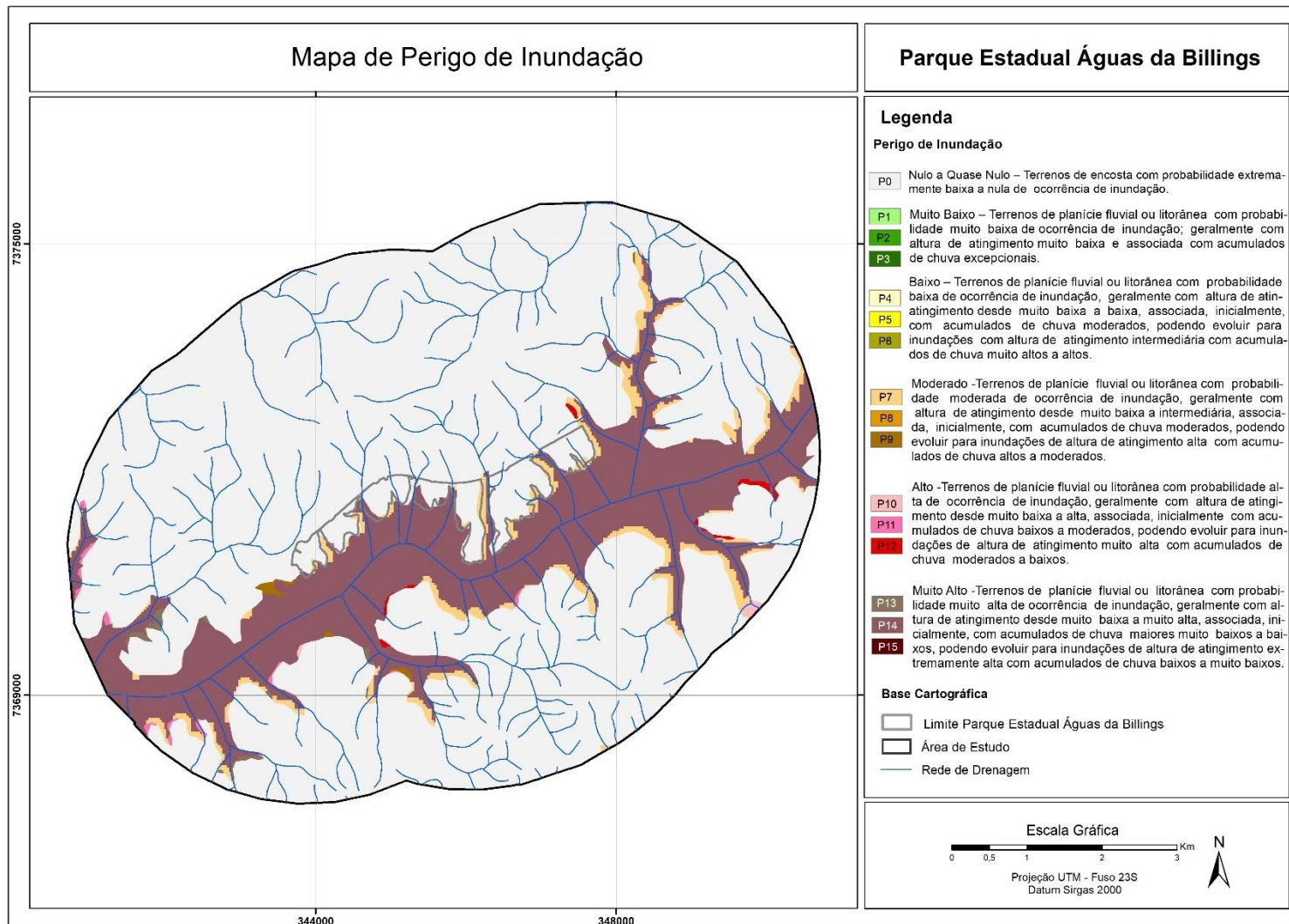
APÊNDICE 3.7.G Mapa de Perigo de Inundação da área de estudo. Fonte: autores.
