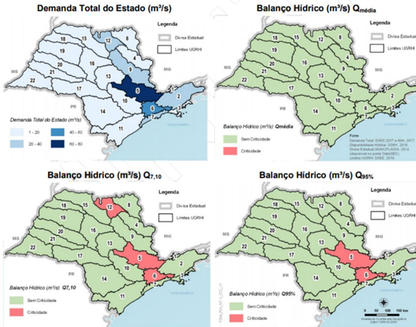
APÊNDICE 3.5.F Criticidade quantitativa da UGRHI 06 em 2017 (Fonte: SÃO PAULO, 2020).
