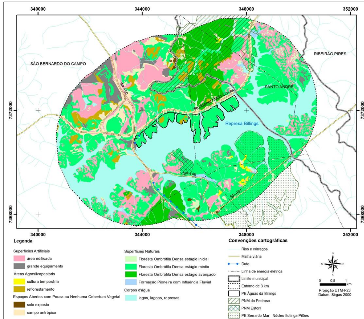
APÊNDICE 3.14.B Mapa de uso e cobertura da terra no entorno de 3km do PE Águas da Billings.
